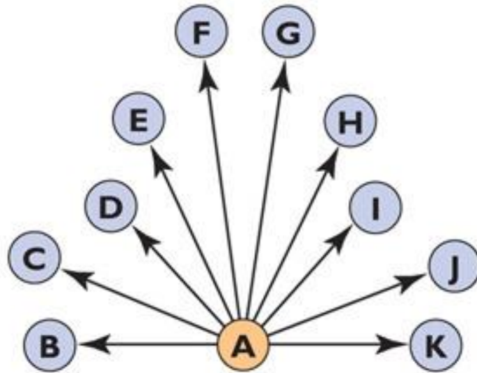
Gossip
